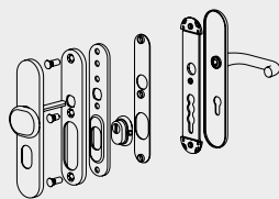
Ferramenta di sicurezza ES 2 Security hardware ES 2
