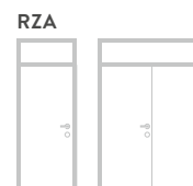
Raumhohe Zarge mit Querteil, Kämpfer und Oberlichte (einflügelig, zweiflügelig)
