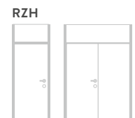
Raumhohe Zarge ohne Querteil mit Kämpfer und Oberlichte (einflügelig, zweiflügelig)
