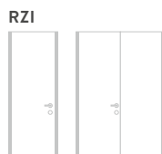
Raumhohe Zarge ohne Querteil und ohne Kämpfer (einflügelig, zweiflügelig)
